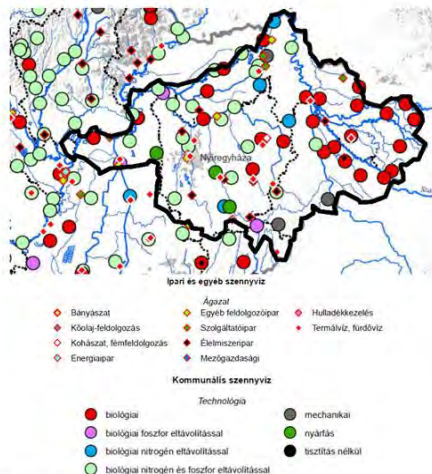
54. ábra: Kommunális és ipari szennyvíz bevezetések
