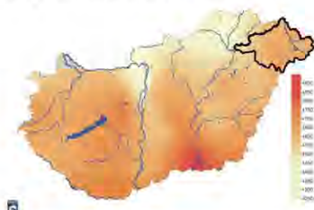
89. ábra: A globálisugárzás (MJ/m 2 ) átlagos évi összege Magyarországon (forrás: www.met.hu)
